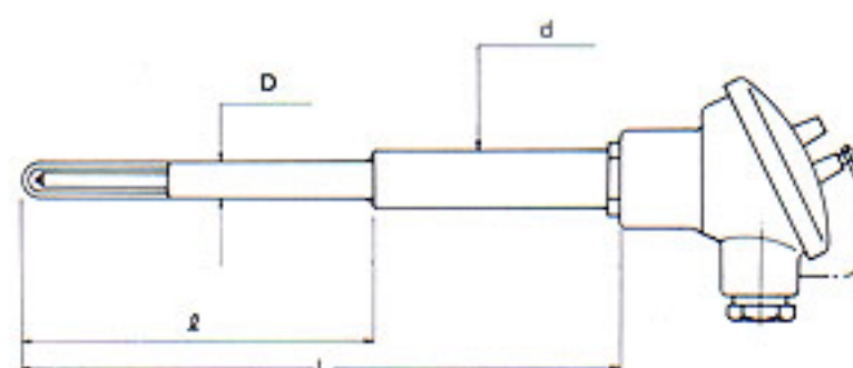
(8) 非金属保護管型
