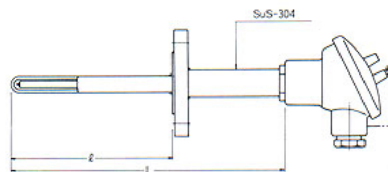
(8) 非金属保護管 固定フランジ型
